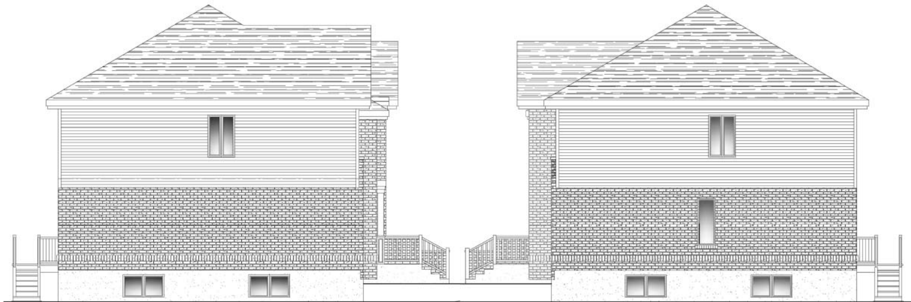
ÉLÉVATION LATÉRALE GAUCHE
